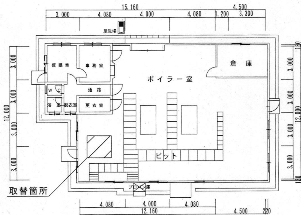
9号建物平面図 S=1:10000
