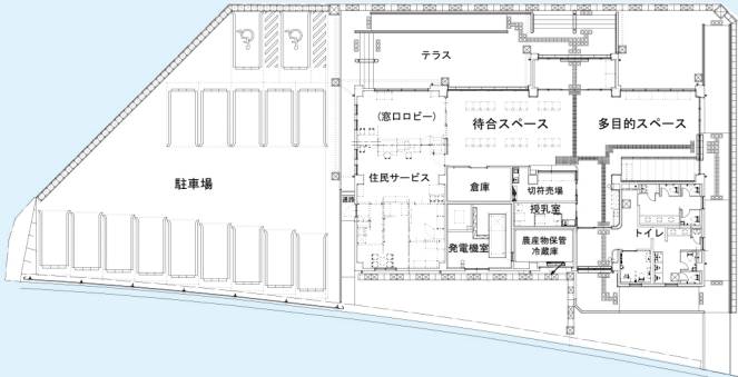
■施設平面図
