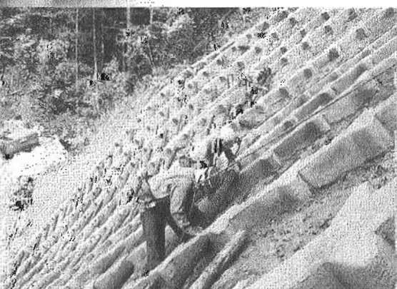
間伐材を有効利用した法面保護工法
