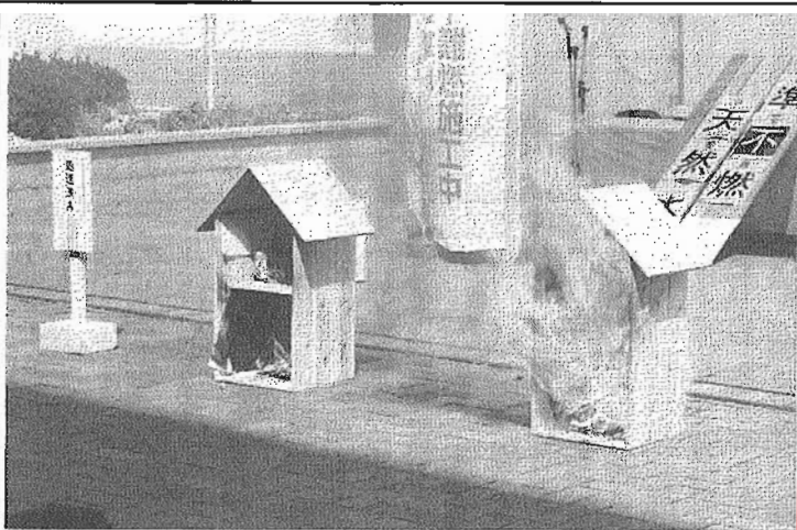
燃焼率の差が歴然とした燃焼実験 ＝北九州市の同会場敷地内で
