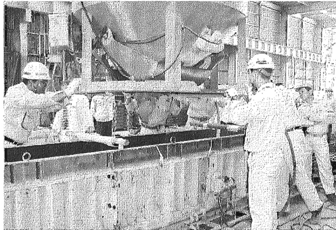
シラスコンクリートの流動性を確認する関係者 ＝鹿児島市東開町で
